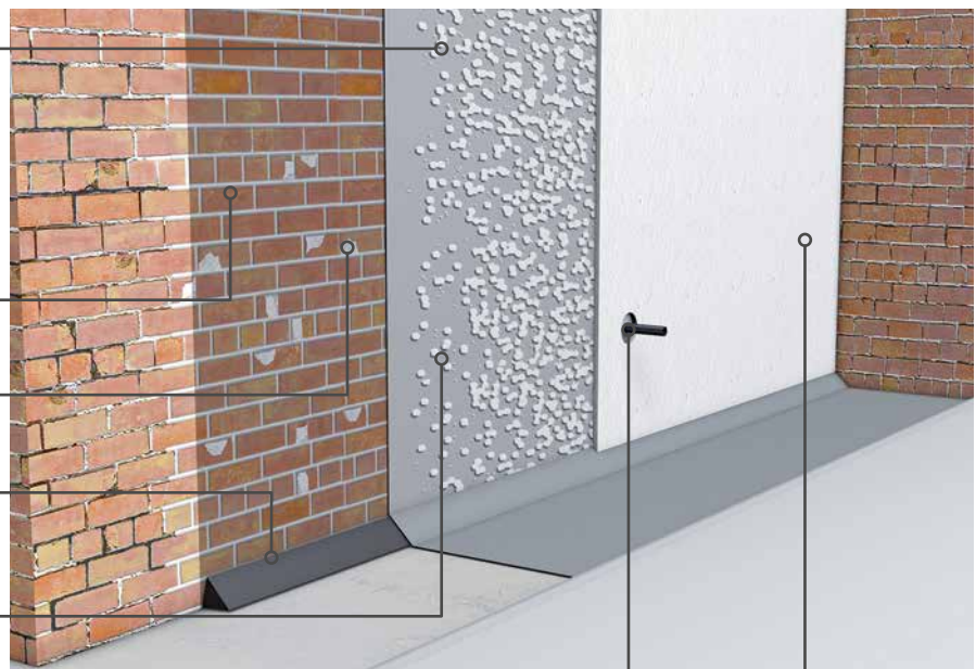
Systeemvoorbeeld
